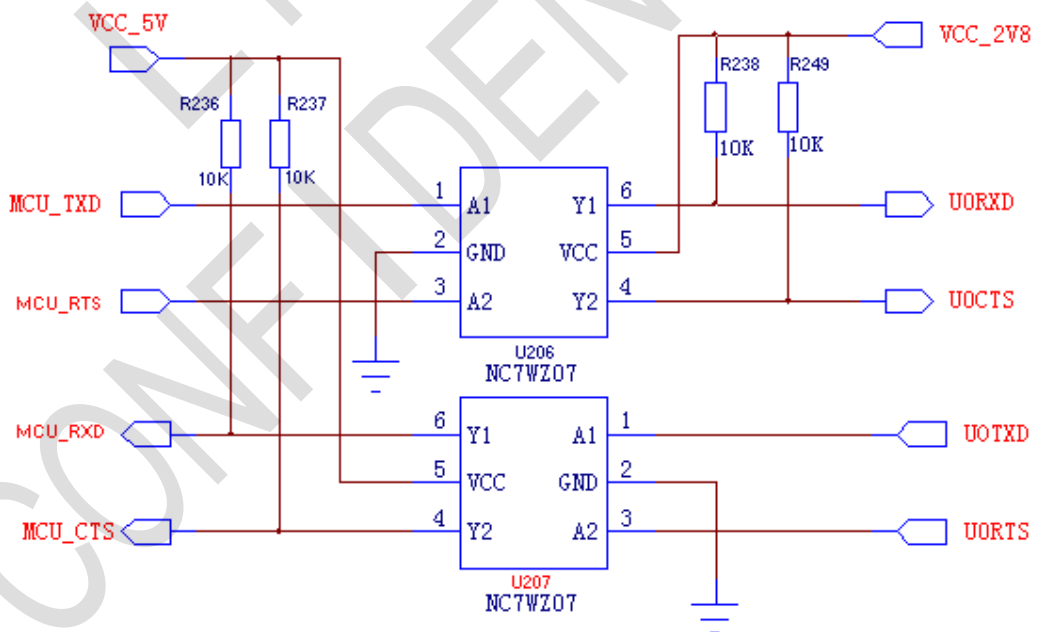
图 3-24: 芯片电平匹配参考电路
