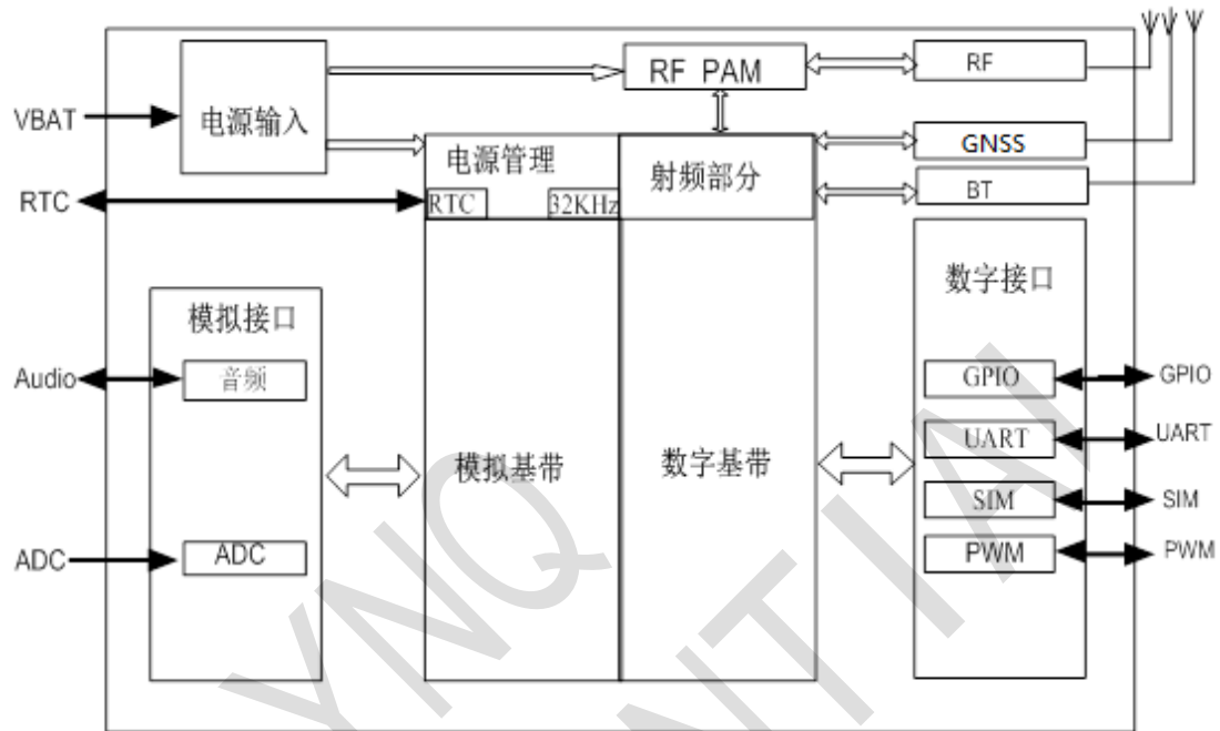
图 1-1: 模块功能框图
