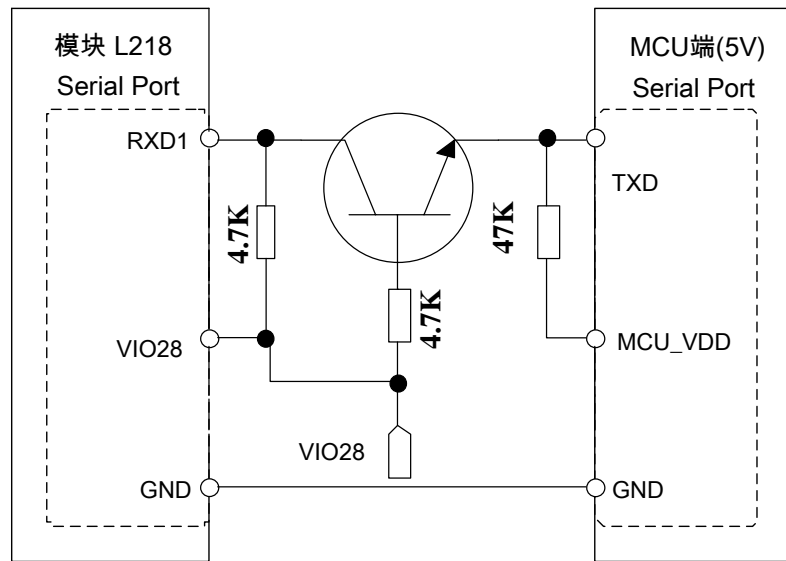
图 3-23: 5V RXD 电平匹配参考电路
