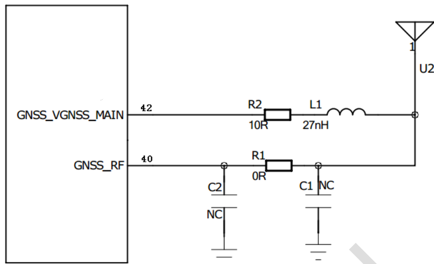
图 3-33: GNSS 有源天线参考电路
