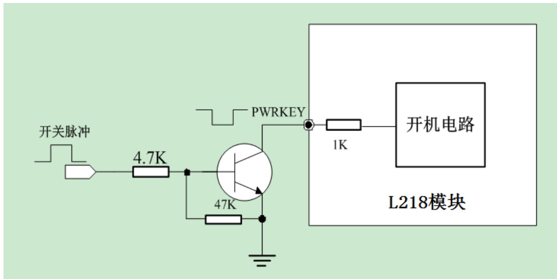
图 3-6: 用三极管控制开机
