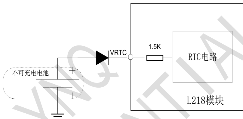
图 3-14: 不可充电电池给 RTC 供电
