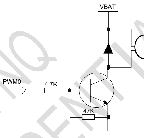
图 3-29: PWM 参考电路
