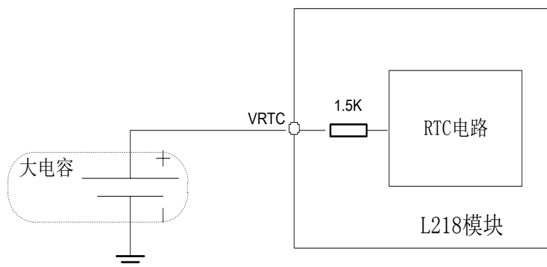
图 3-13: 外部电容给 RTC 供电
