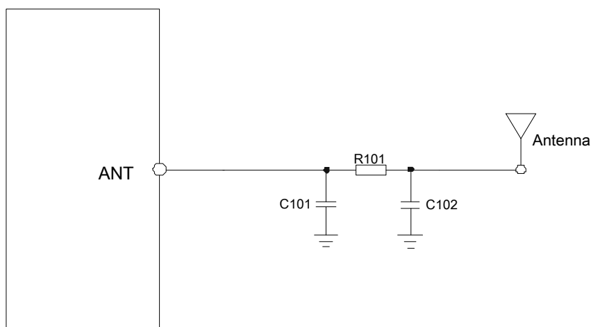
图 3-31: 射频参考电路 (GSM /BT)
