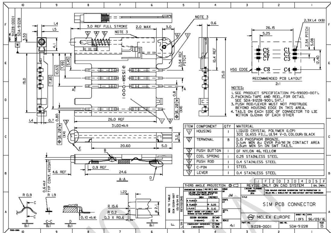
图 3-27: Molex 91228 SIM 卡座
