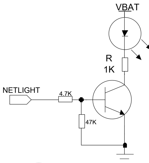
图 3-30: NETLIGHT 参考设计电路
