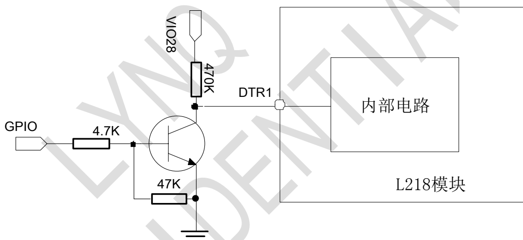
图 3-12: DTR 脚的控制示意
