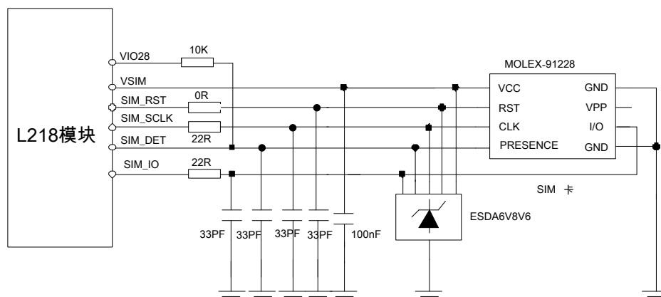
图 3-25: 8-pin SIM 卡参考电路
