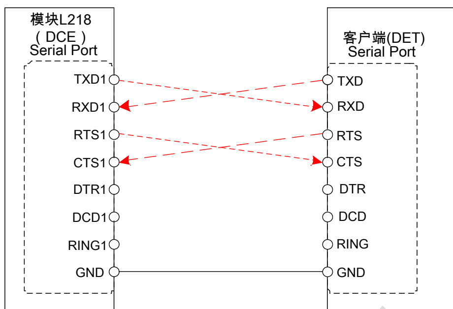
图 3-20:串口带流控连接示意
