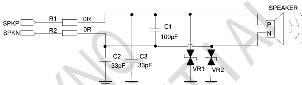
图 3-16: 喇叭参考电路
