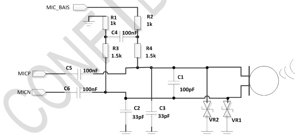
图 3-17: 麦克风参考电路
