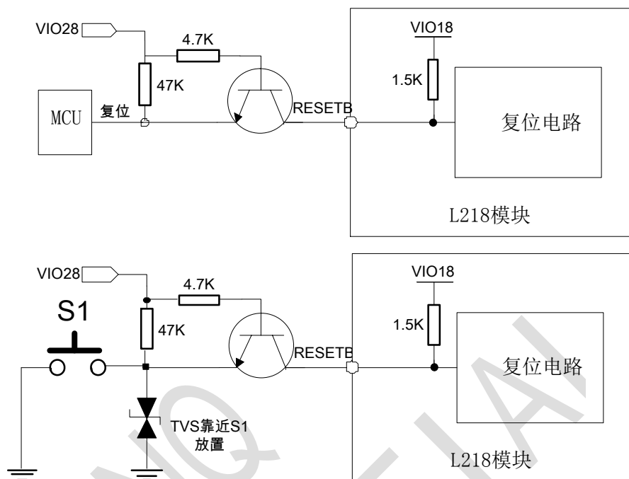
图 3-10: 推荐复位电路
