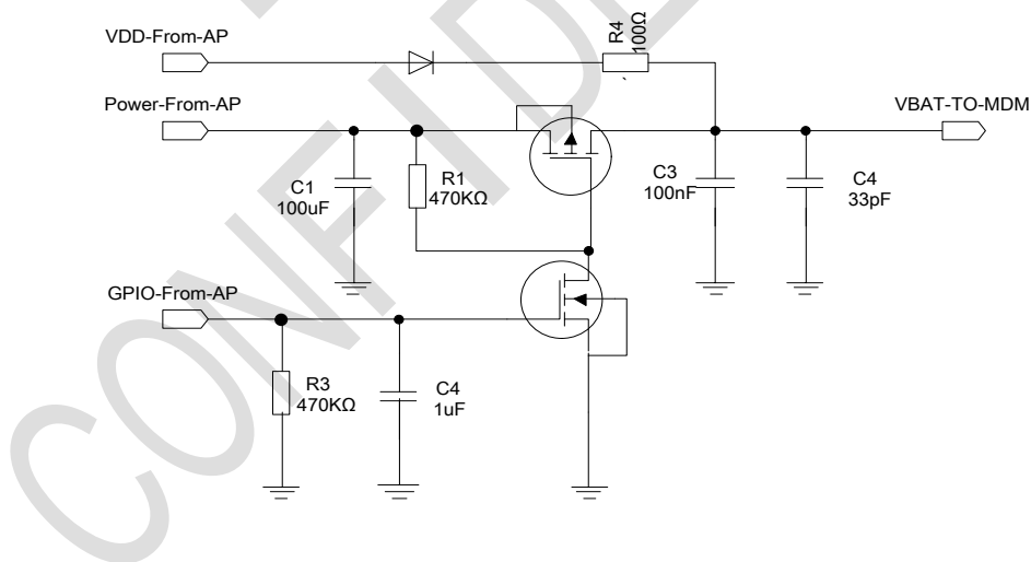
图 3-5: PMOS 控制参考电路（仅供参考）
