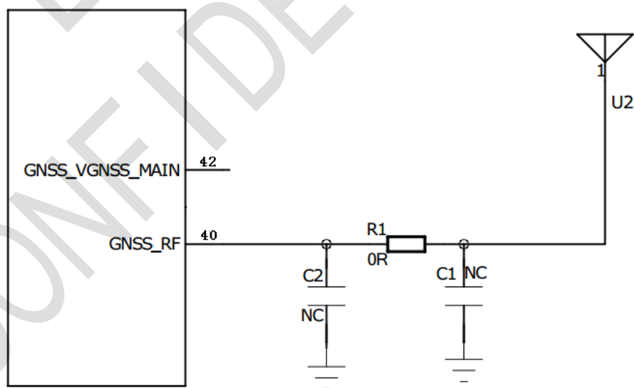
图 3-32: GNSS 无源天线参考电路
