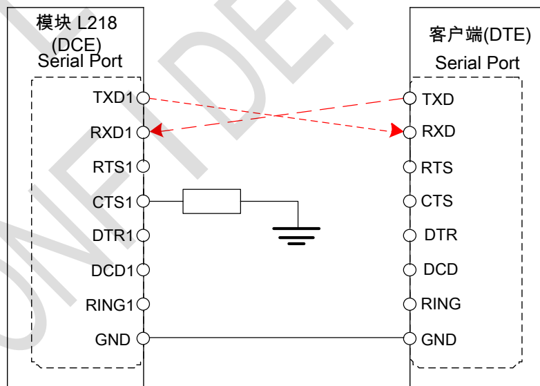
图 3-19:串口三线连接示意
