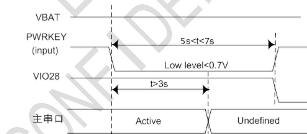
图 3-9: 关机时序
