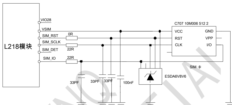
图 3-25: 8-pin SIM 卡参考电路
