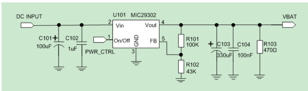
图 3-3: LDO 参考电路(仅供参考)
