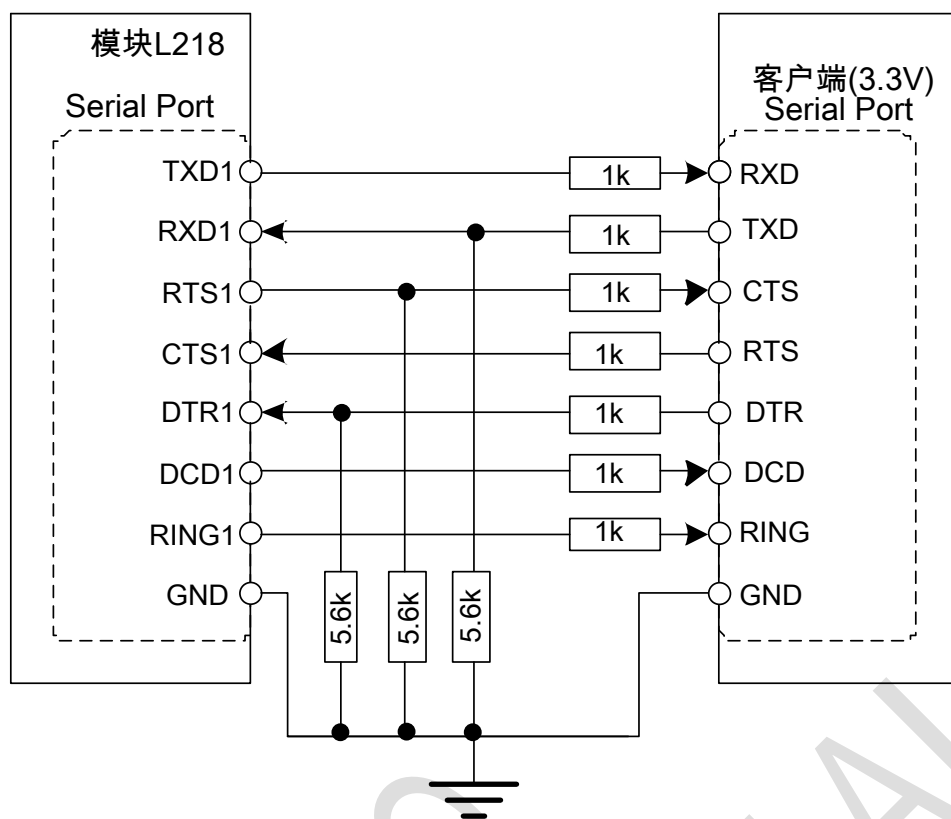
图 3-21:电阻电平匹配参考电路
