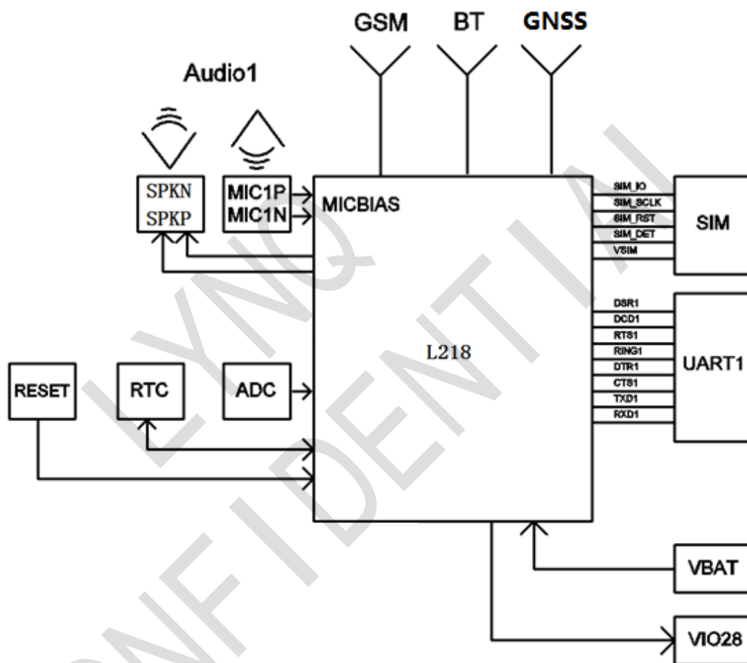
图 4-2: 系统功能框图
