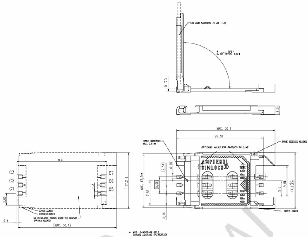
图 3-28: Amphenol C707 10M006 5122 SIM 卡座尺寸图
