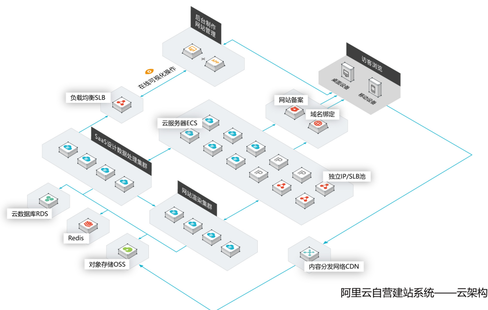
(架构图)
